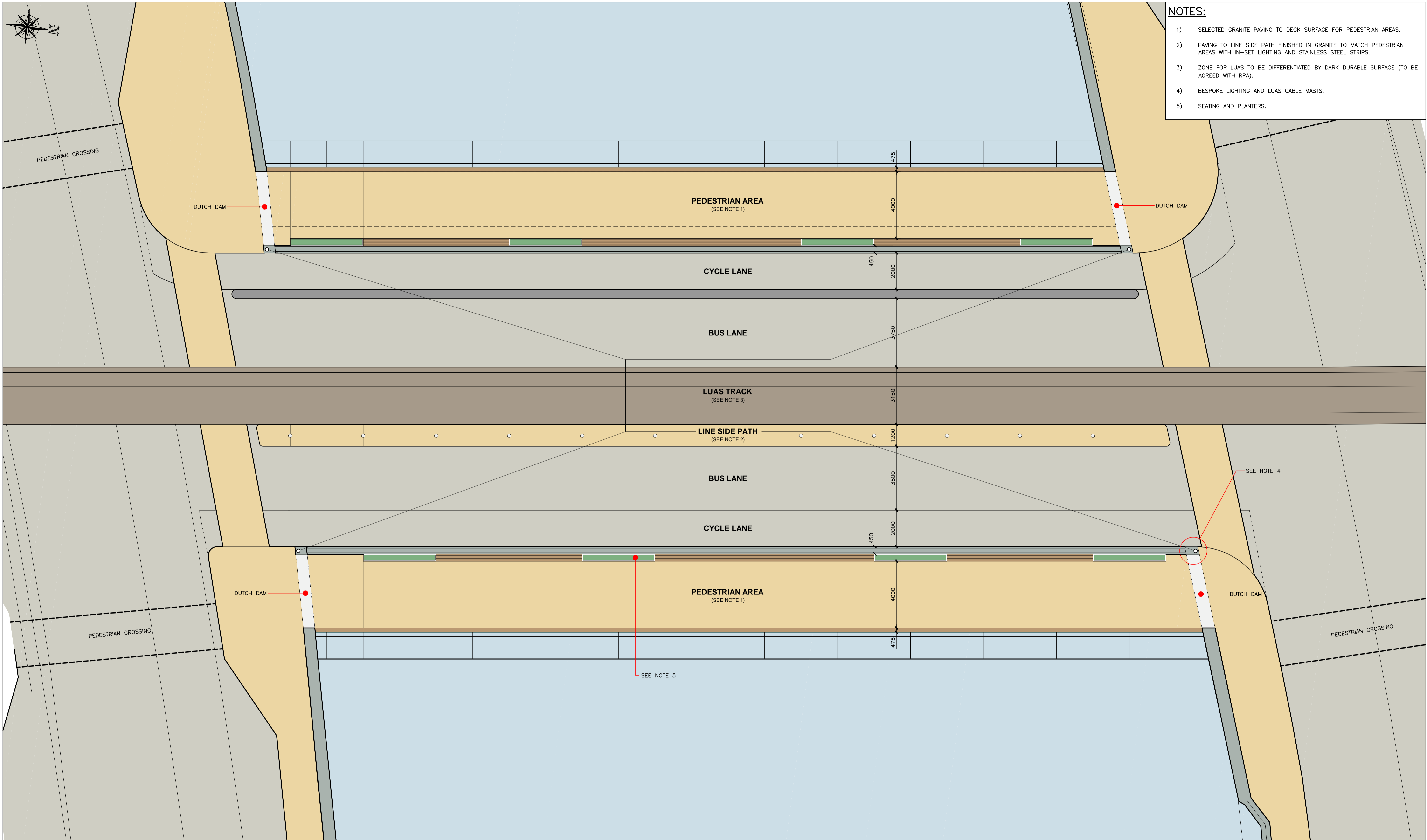
PLAN A1 SCALE 1:100 A3 SCALE 1:200
